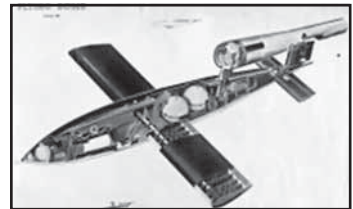
220 V1 - cutaway
